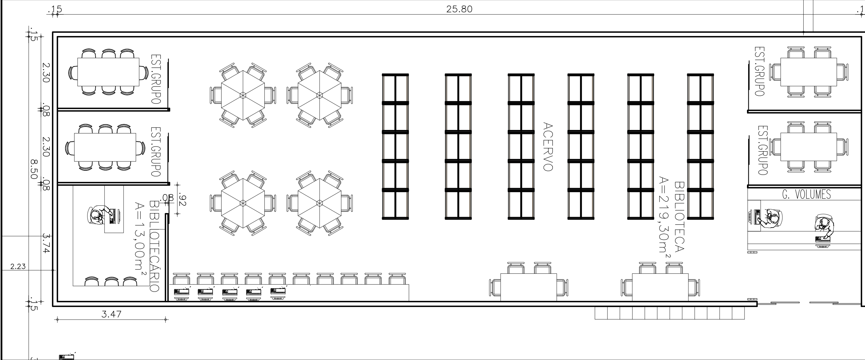
PLANTA - BIBLIOTECA UNINTA ITAPIPOCA BLOCO 04
